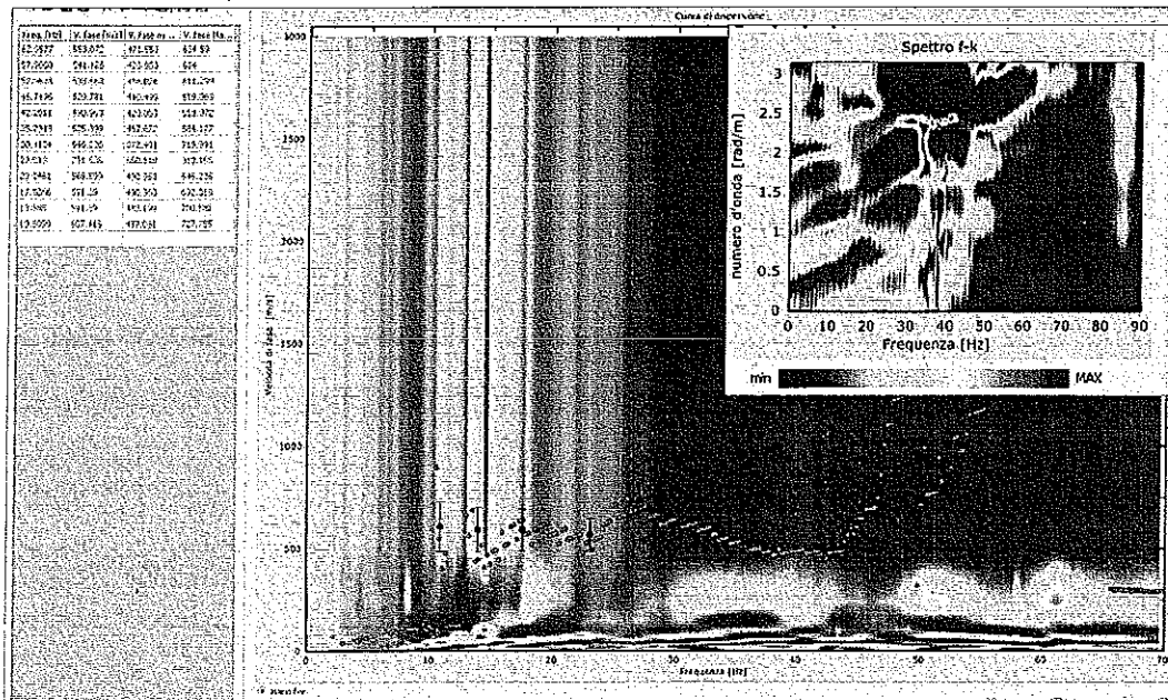
Figura 3: Curva di dispersione e spettro f-k
