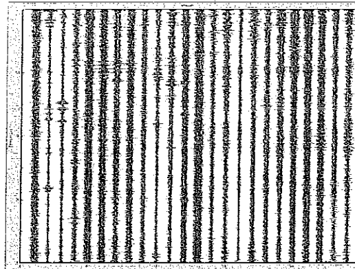
Figura 2: Tracce sperimentali tecnica passiva REMI
